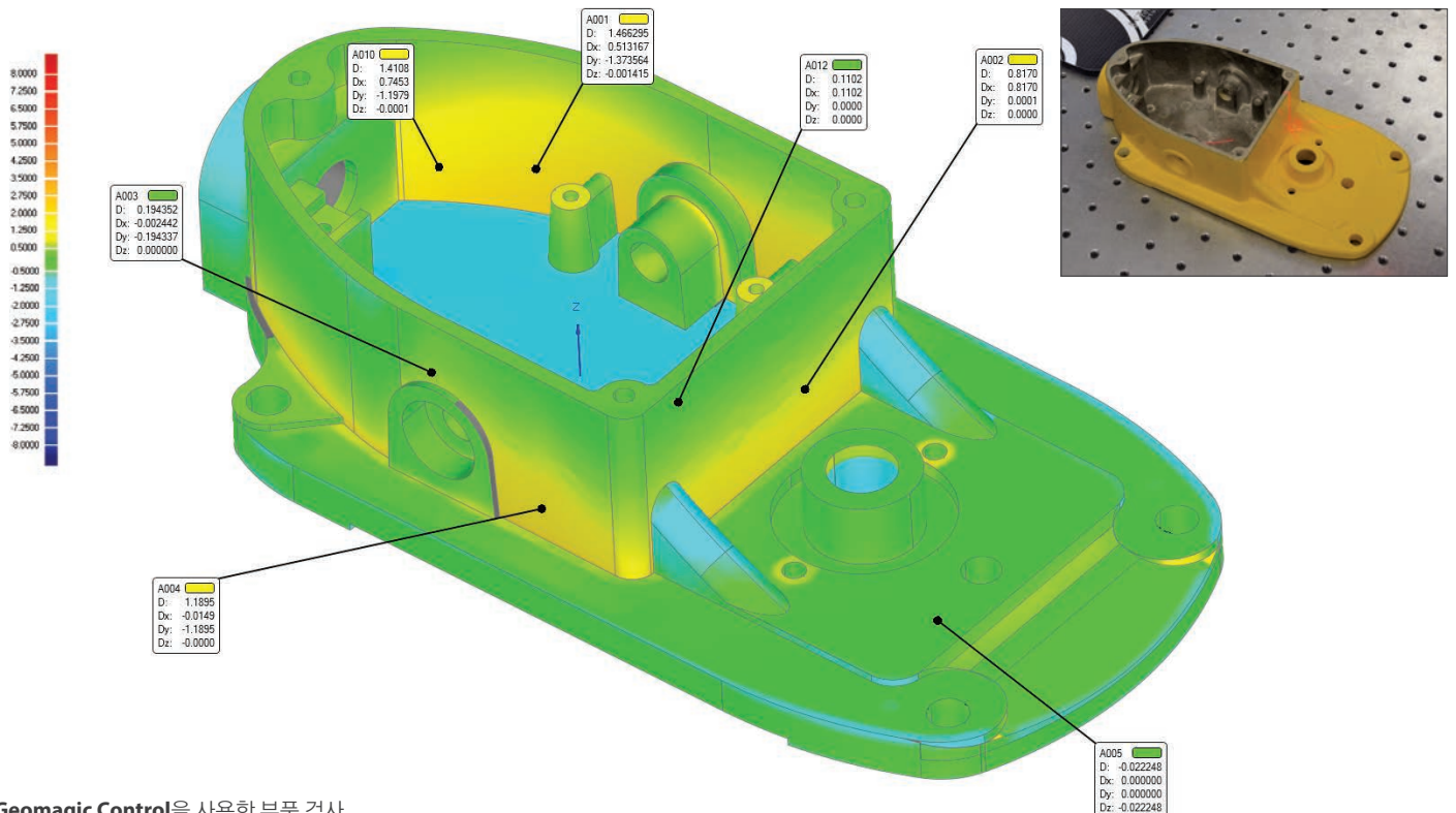
Geomagic Control을 사용한 부품 검사
